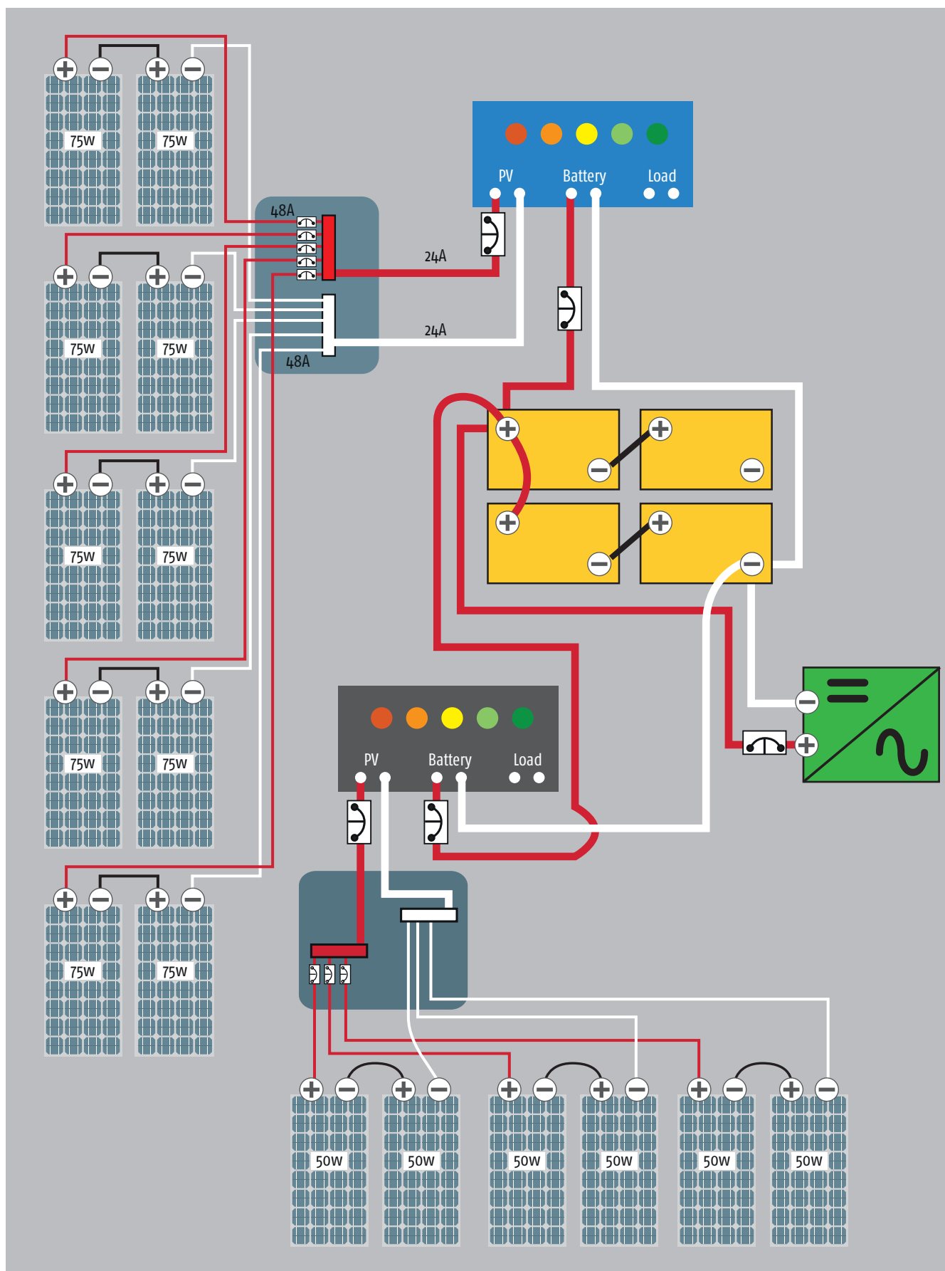
Figura 11. Configuración del sistema fotovoltaico para la Unidad Educativa de Carmen del Emero
