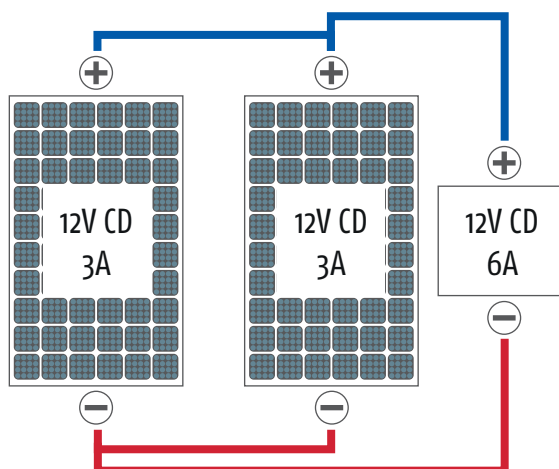
Figura 8. Módulos conectados en paralelo
