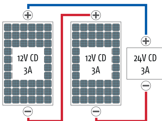
Figura 7. Módulos conectados en serie
