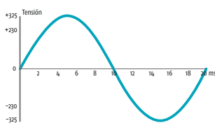
Fig 4. Representación gráfica de CA
