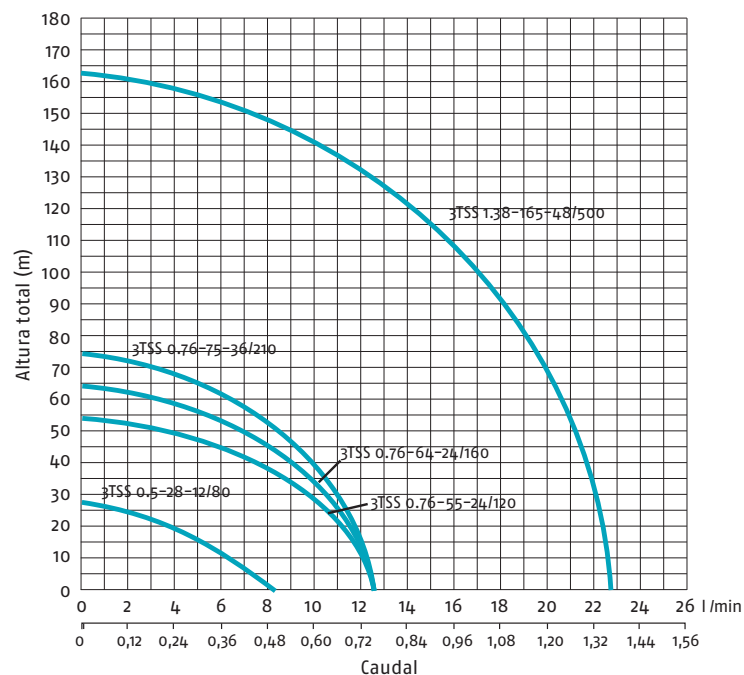
Figura 13: Grafico del funcionamiento de la bomba
