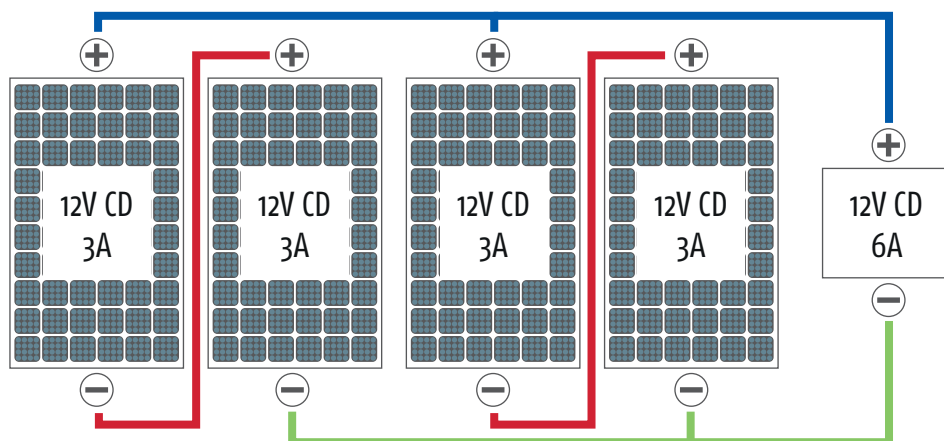
Figura 9. Módulos conectados en serie y en paralelo
