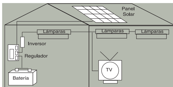
Figura 2. Esquema simple de un sistema fotovoltaico
