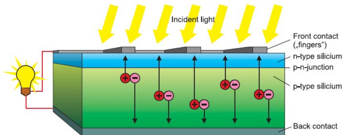
Figura 2: vista general esquemática del proceso en una célula fotovoltaica 1
