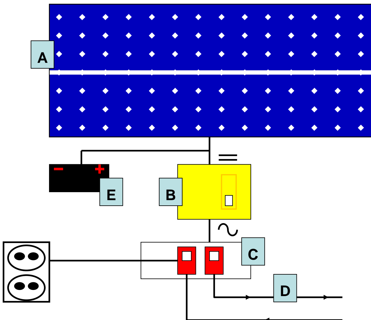
Figura 3: descripción general de un sistema FV 2
