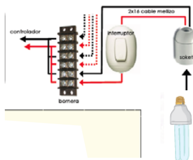
Ilustración 10 Esquema de conexiones de soket a bornera de baquelita
