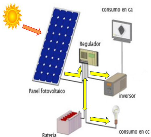
Ilustración 4 Sistema fotovoltaico típico
